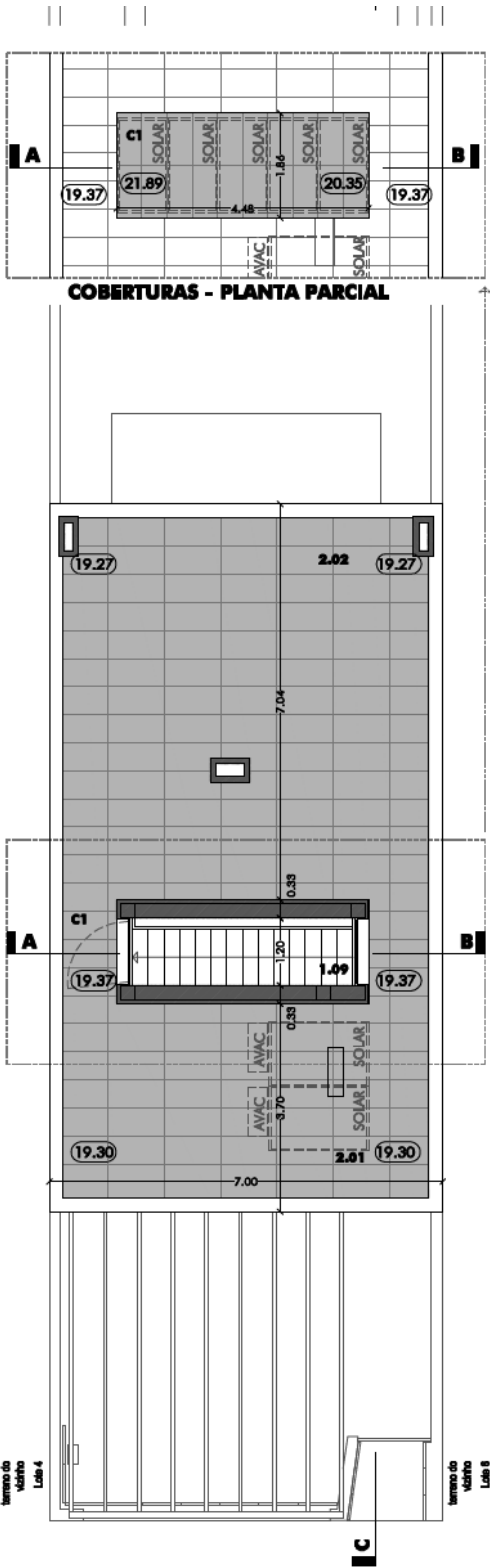
Lote 8 Planta do Piso de Cobertura
