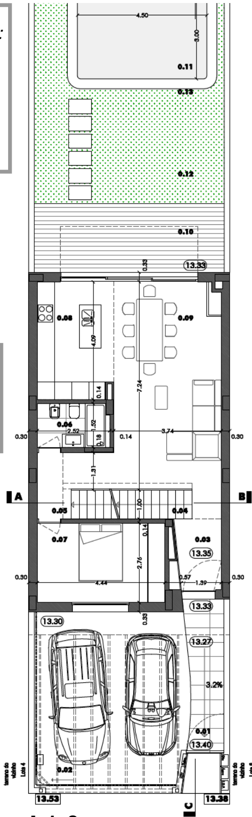
Lote 8 Planta do Piso 0
