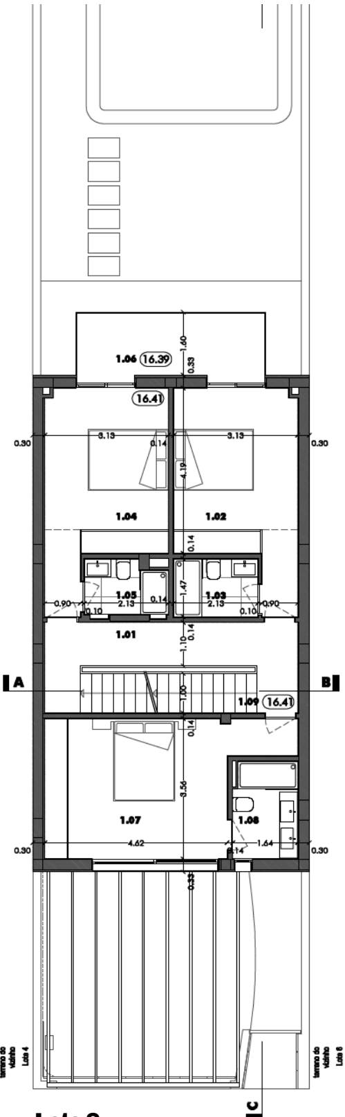
Lote 8 Planta do Piso 1
