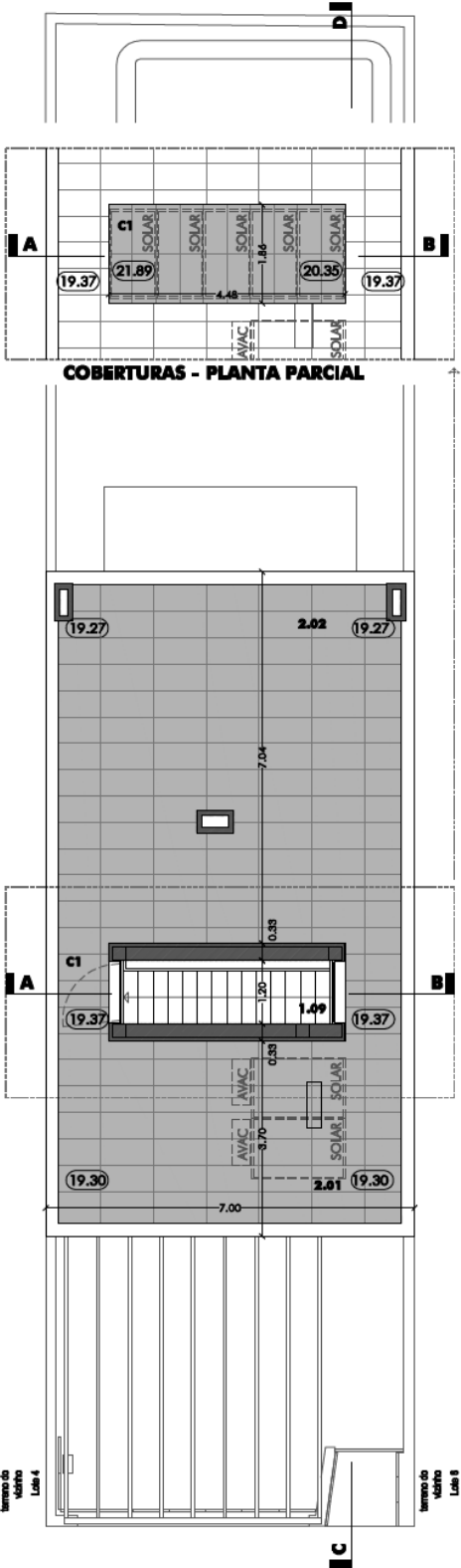
Lote 7 Planta do Piso de Cobertura
