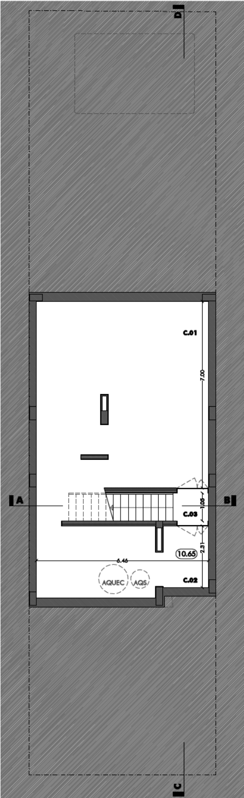
Lote 7 Planta da Cave
