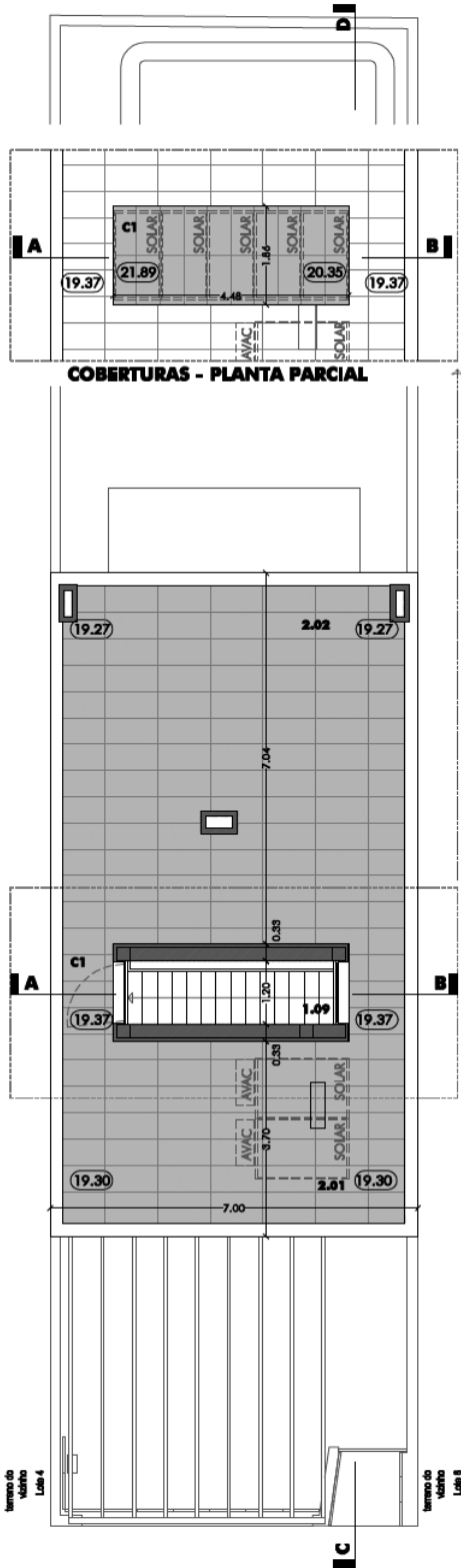
Lote 6 Planta do Piso de Cobertura
