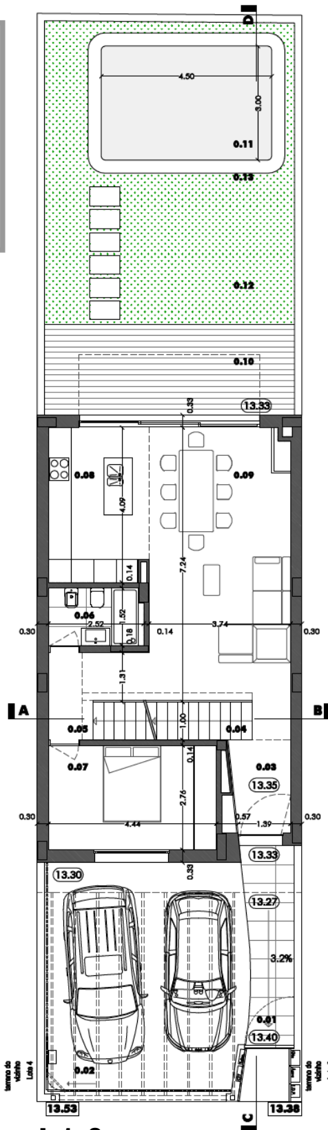
Lote 6 Planta do Piso 0
