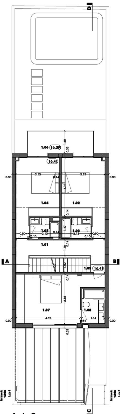
Lote 6 Planta do Piso 1
