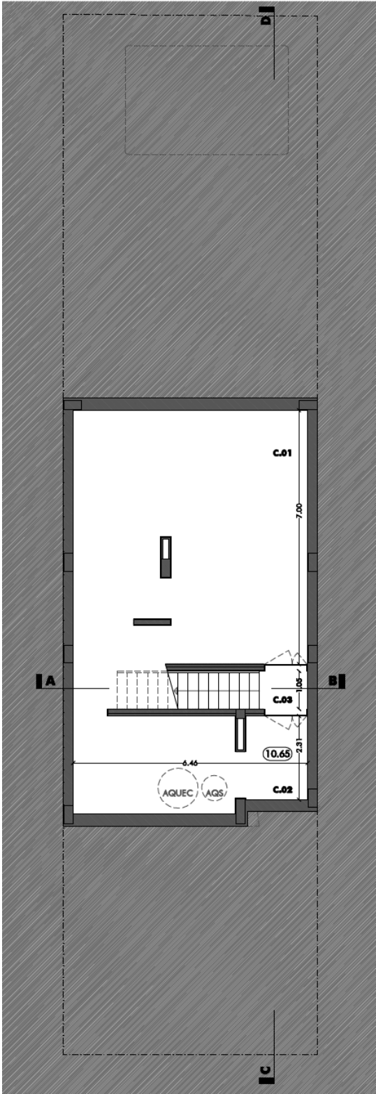
Lote 6 Planta da Cave
